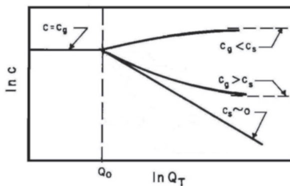
شکل ۲: نمودار لگاریتم غلظت TDS برحسب لگاریتم جریان
