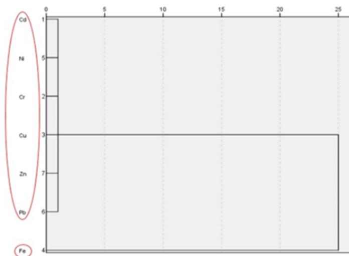
شکل ۲- نمودار تحلیل خوشه‌ای بر اساس روش Ward
