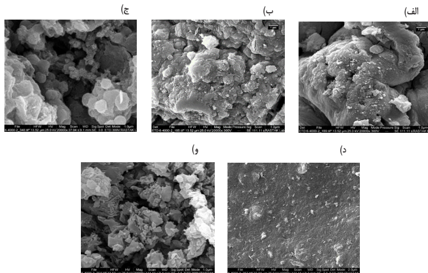
شکل ۲- تصاویر SEM مربوط به گرانول‌های Alg/Fe-Clin تهیه شده در سه نوع محلول اتصال دهنده عرضی مختلف (شامل الف) CaCl_2 ، ب) FeCl_3 + CaCl_2 ، ج) FeCl_3 و گرانول‌های CS/Fe-Clin تهیه شده در دو نوع محلول اتصال دهنده عرضی شامل د) STPP و STPP + NaOH
