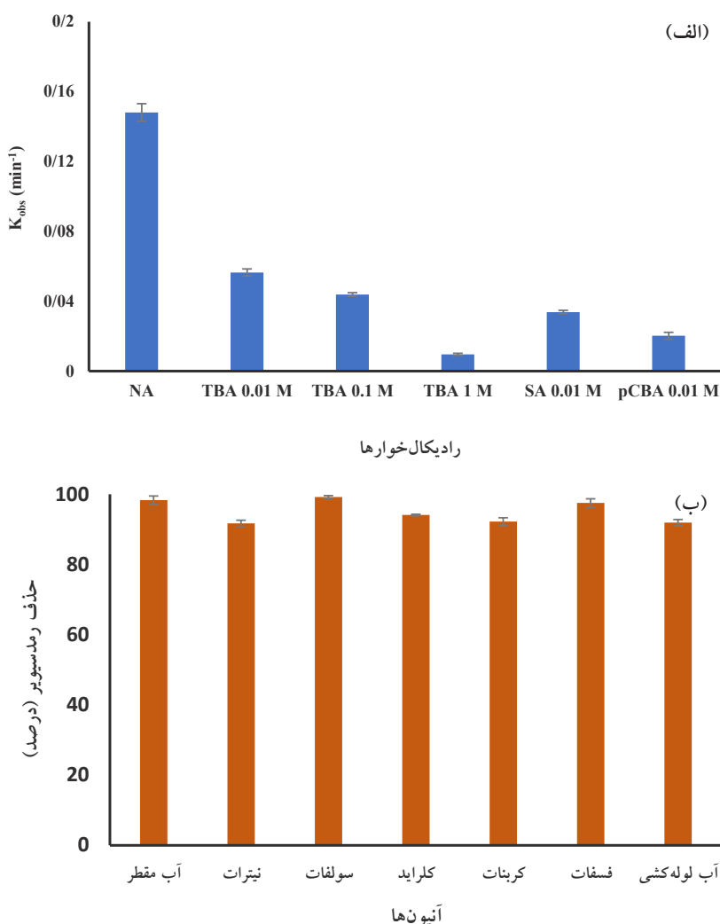
نمودار ۵- اثر رادیکال‌خوارها بر فرایند تجزیه VUV/H_2O_2 (الف) ثابت سرعت تجزیه فرآیند VUV/H_2O_2 و (ب) اثر غلظت ۱ mM آنیون‌ها بر راندمان حذف رمدسیویر (غلظت رمدسیویر ۲۰ mg/L و pH برابر با ۷)
