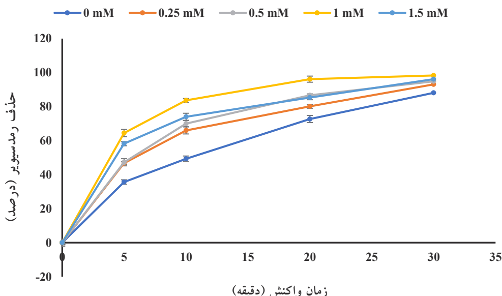
نمودار ۴- اثر غلظت H_2O_2 بر کارایی فرآیند VUV در تجزیه رمدسیویر ۲۰ mg/L و زمان ۳۰ min و pH برابر ۷
