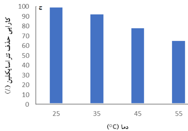
نمودار ۲- (الف) اثر دوز جاذب، (ب) اثر زمان تماس و (ج) اثر دما بر کارایی حذف داروی تتراسایکلین توسط گرافن اکساید مغناطیسی عامل دار شده با \beta سیکلودکستین
