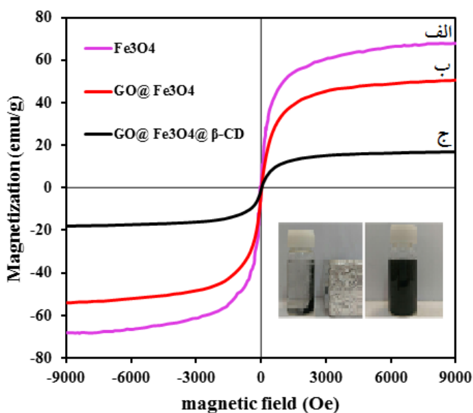
شکل ۴- منحنی VSM مگنتایت (الف)، گرافن اکساید مغناطیسی (ب) و گرافن اکساید مغناطیسی عامل دار شده با \beta سیکلودکسترین (ج)
