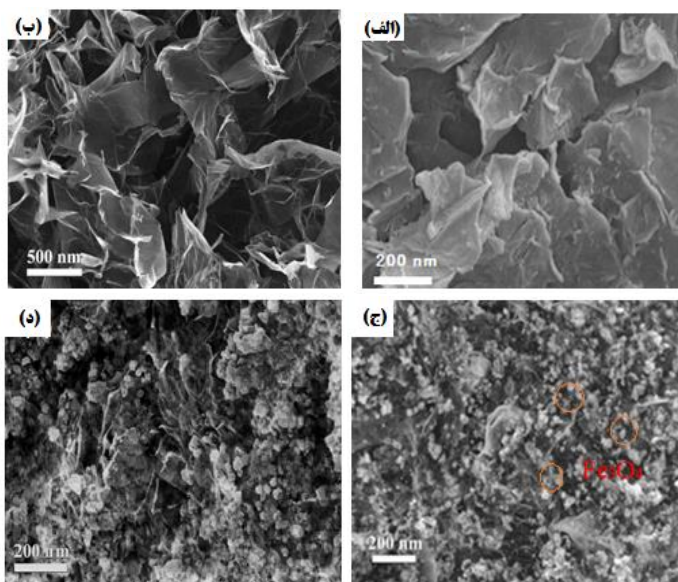
شکل ۱- تصویر SEM از گرافن (الف)، گرافن اکساید (ب)، گرافن اکساید مغناطیسی (ج)، و گرافن اکساید مغناطیسی عامل‌دار شده با \beta سیکلودکسترین (د)
