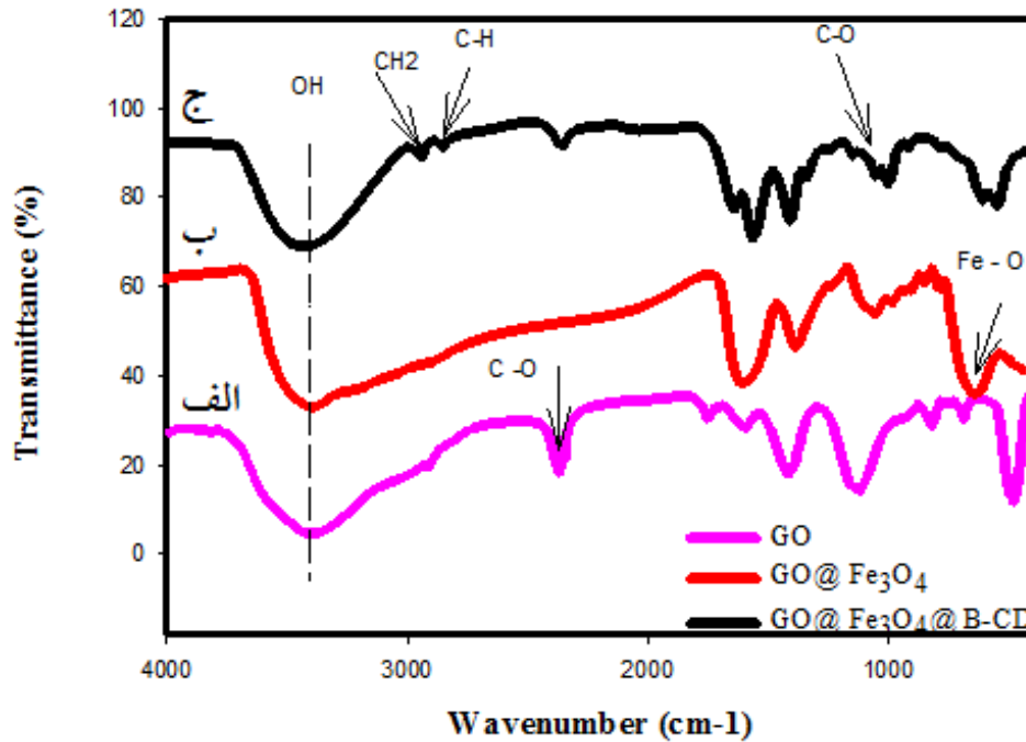
شکل ۳- طیف FT-IR از گرافن اکساید (الف)، گرافن اکساید مغناطیسی (ب) و گرافن اکساید مغناطیسی عامل‌دار شده با \beta سیکلودکسترین (ج)
