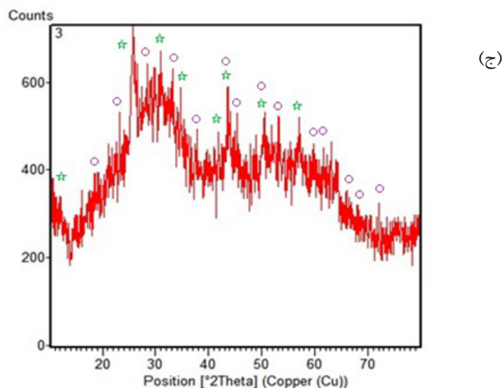
ادامه شکل ۲- نتایج آنالیز XRD نمونه‌های (الف) PMo، (ب) UiO-66 و (ج) PMo/UiO-66
