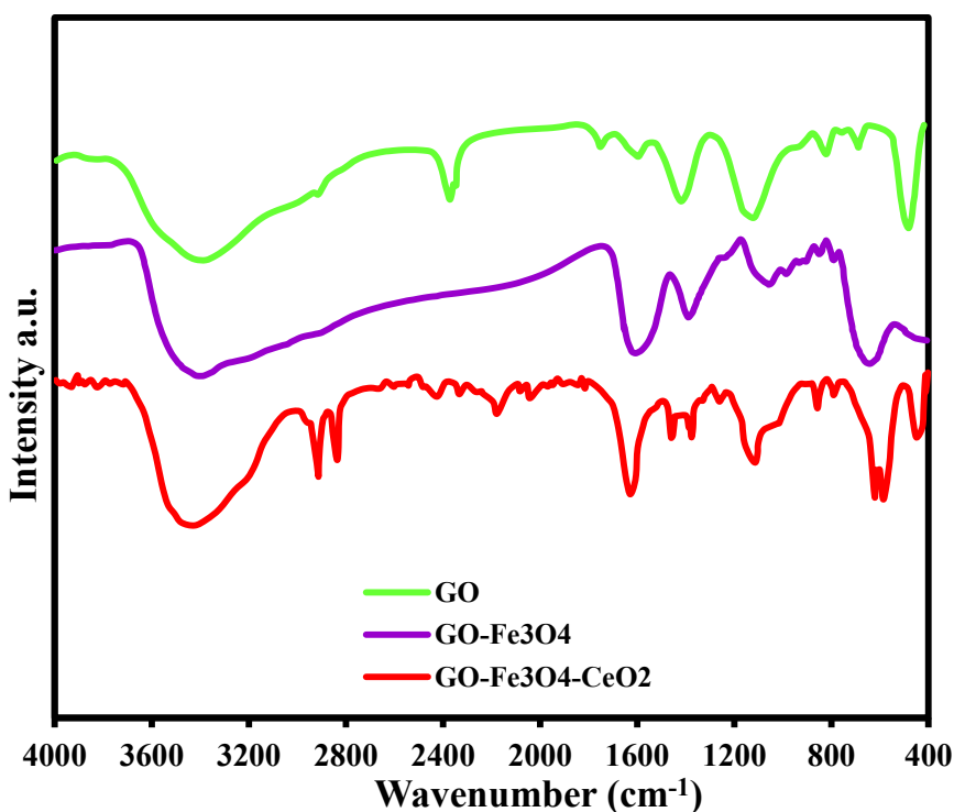
شکل ۴- تصویر FTIR از گرافن اکساید، گرافن اکساید مغناطیسی، گرافن اکساید مغناطیسی عامل دار شده با دی اکسید سریم
