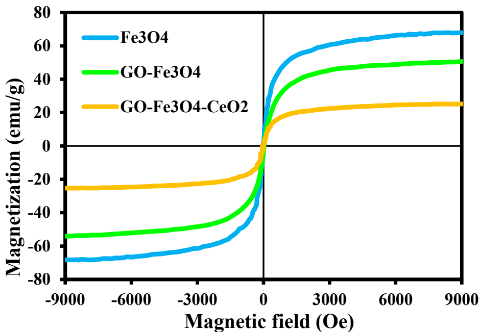
شکل ۵- تصویر VSM از گرافن اکساید، گرافن اکساید مغناطیسی، گرافن اکساید مغناطیسی عامل دار شده با دی اکسید سریم
