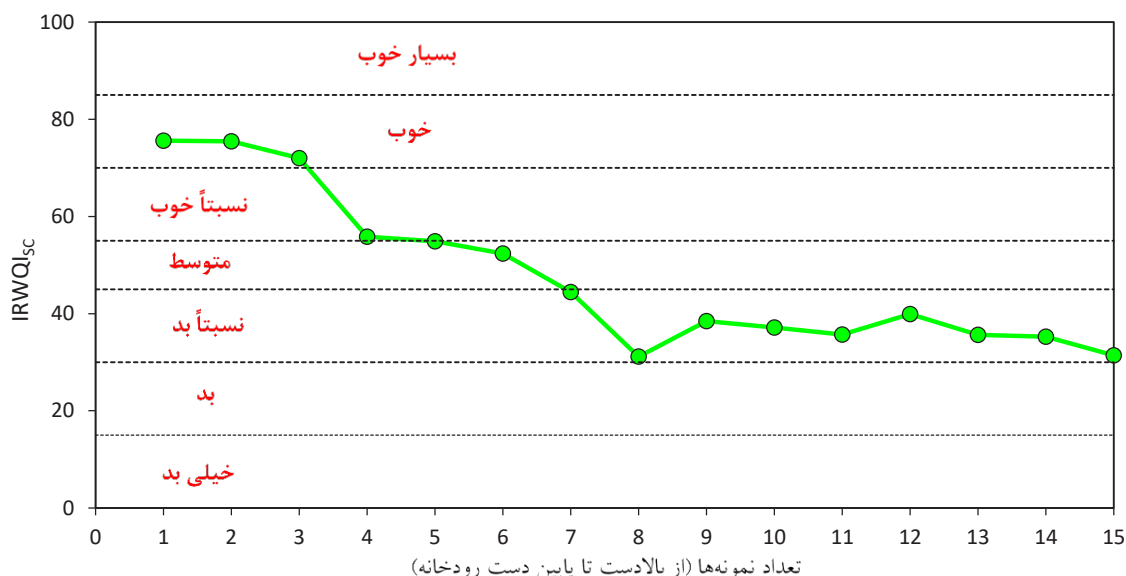
نمودار ۲- شاخص IRWQI_{sc} در ایستگاه‌های نمونه‌برداری طول رودخانه مه‌باد
