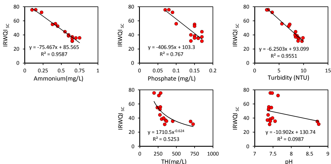
ادامه نمودار ۳- ارتباط بین شاخص IRWQI sc با پارامترهای فیزیکی و شیمیایی آب
