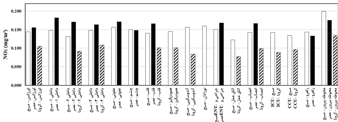
NO 2 (mg/m 3 ) - میانگین
