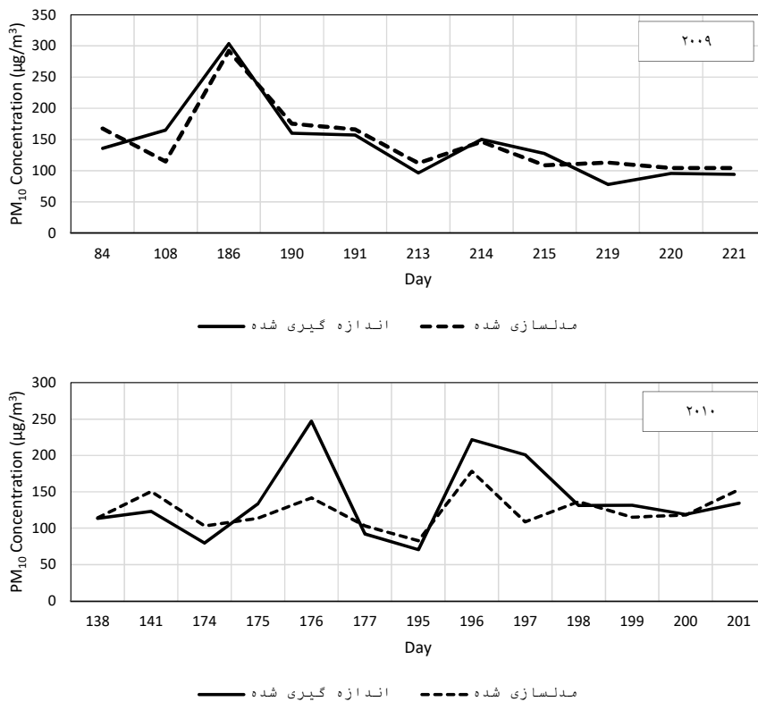
ادامه نمودار ۳- تغییرات روزانه PM_{10} اندازه‌گیری شده و مدل‌سازی شده مربوط به سال ۲۰۰۸، ۲۰۰۹ و ۲۰۱۰
