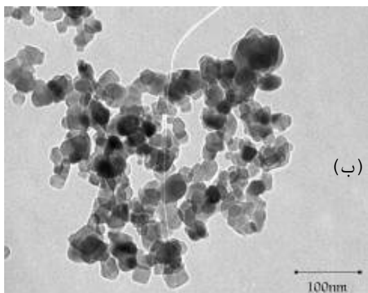
شکل ۱- شمای فتوراکتور (a) کپسول اکسیژن، (b) مانومتر، (c) شیلنگ، (d) لامپ UV-C، (e) راکتور لوله‌ای کوارتز، (f) پایه، (g) محفظه چوبی (الف) و تصویر TEM از نانوذرات TiO_2 (ب)
