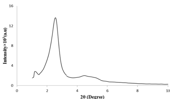
شکل ۳- طیف XRD مربوط به MCM-41
