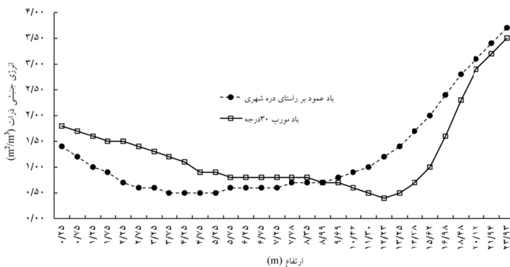
نمودار ۳- ضریب جابجایی آشفته ذرات آلاینده در دو جهت وزش باد دره شهری
