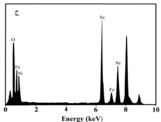
شکل ۲- (الف) تصویر TEM از نانوذرات مغناطیسی نیکل، (ب) طیف XRD بدست آمده از نانوذرات مغناطیسی نیکل، (ج) آنالیز EDX از نانوذرات مغناطیسی نیکل
