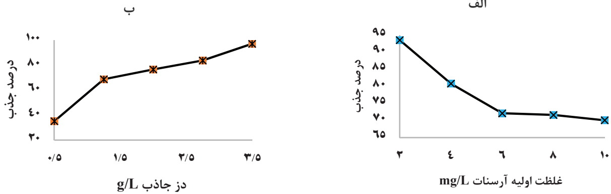
شکل ۴- تاثیر غلظت‌های مختلف آرسنات (ج) و جاذب (د) بر میزان جذب آرسنات توسط جاذب nZVI-Chitosan در pH=7/5 و زمان تماس 91/25 min
