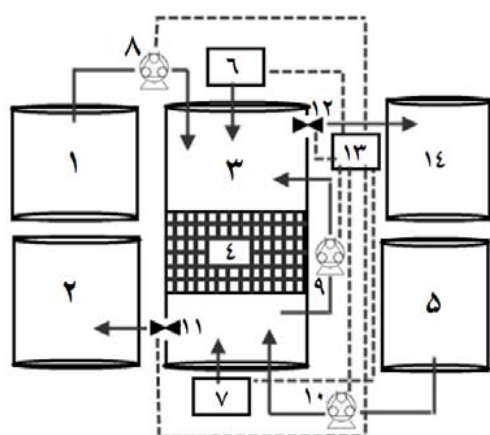
شکل ۲- شکل شماتیک پایلوت؛ (۱) مخزن خوراک، (۲) مخزن پساب، (۳) راکتور بیوفیلمی بستر ثابت، (۴) بستر مدای ثابت، (۵) مخزن شستشوی معکوس، (۶ و ۷) پمپ هوا، (۸ و ۹ و ۱۰) پمپ پرستالتیک، (۱۱ و ۱۲) شیر برقی، (۱۳) تایمرها، (۱۴) مخزن خروجی شستشوی معکوس
