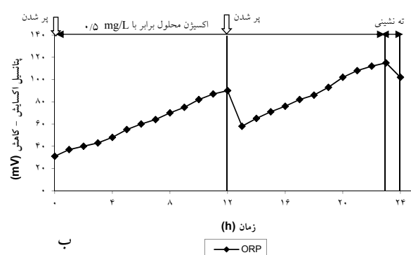
نمودار ۳- الف) تغييرات فرم‌های نيتروژن، ب) تغييرات ORP در يك سيکل از راکتور SBBR در پريود دوم
