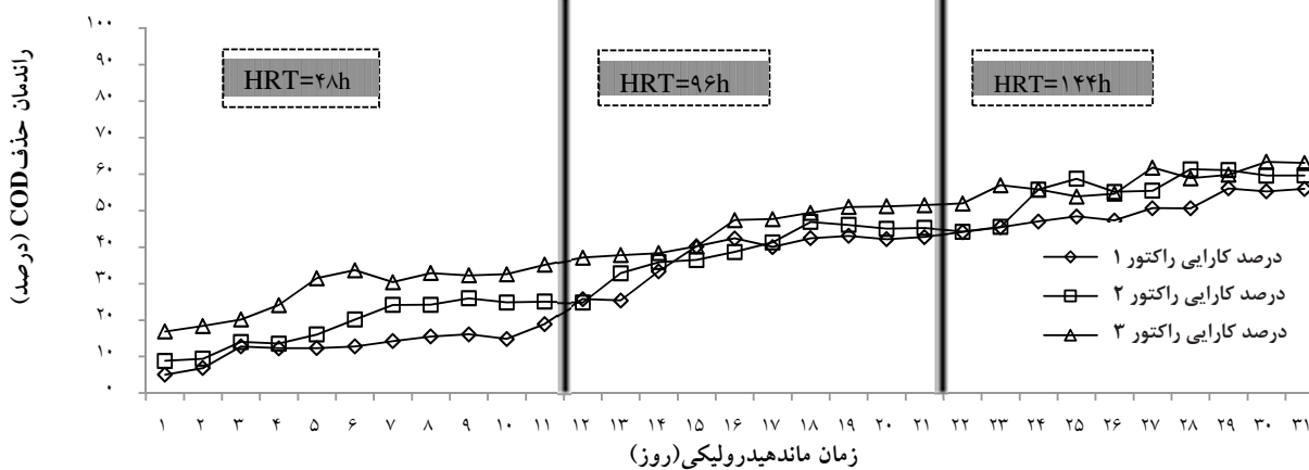
نمودار ۲- تاثیر زمان ماندهای هیدرولیکی و غلظت‌های مختلف پودر کربن فعال در حذف COD
