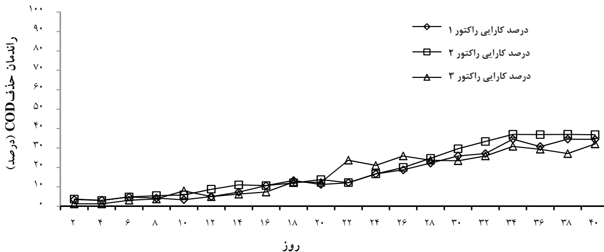
نمودار ۱- کارایی راکتورهای SBR در حذف COD طی مرحله سازگاری باکتری‌ها
