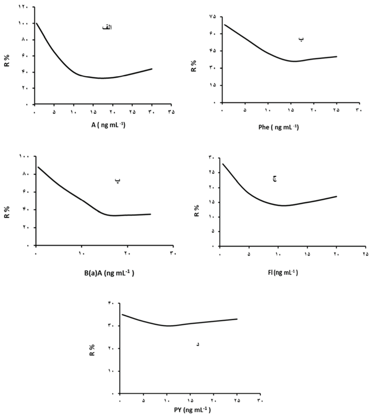
شکل ۴: متحنی کالیبراسیون (الف) آنتراسن (ب) فناترن (پ) بنز (a) آنتراسن (ج) فلورن (د) پیرن در شرایط بهینه بر اساس %R نسبت به غلظت PAHs.
