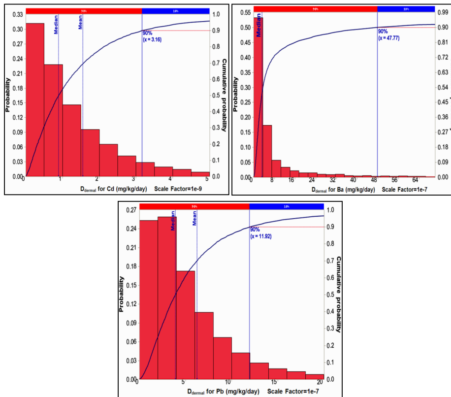
شکل ۱- نمودار توزیع احتمال D_{dermal} برای عناصر Cd، Ba و Pb
