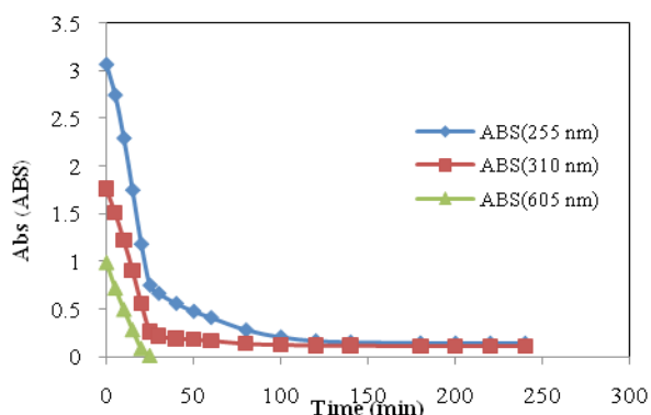
نمودار ۱- نحوه رنگبری رنگزا در شرایط بهینه ( C=100 ppm و P_{UV}=150 W و pH=9 و C_{H_2O_2}=0.1 mM )
