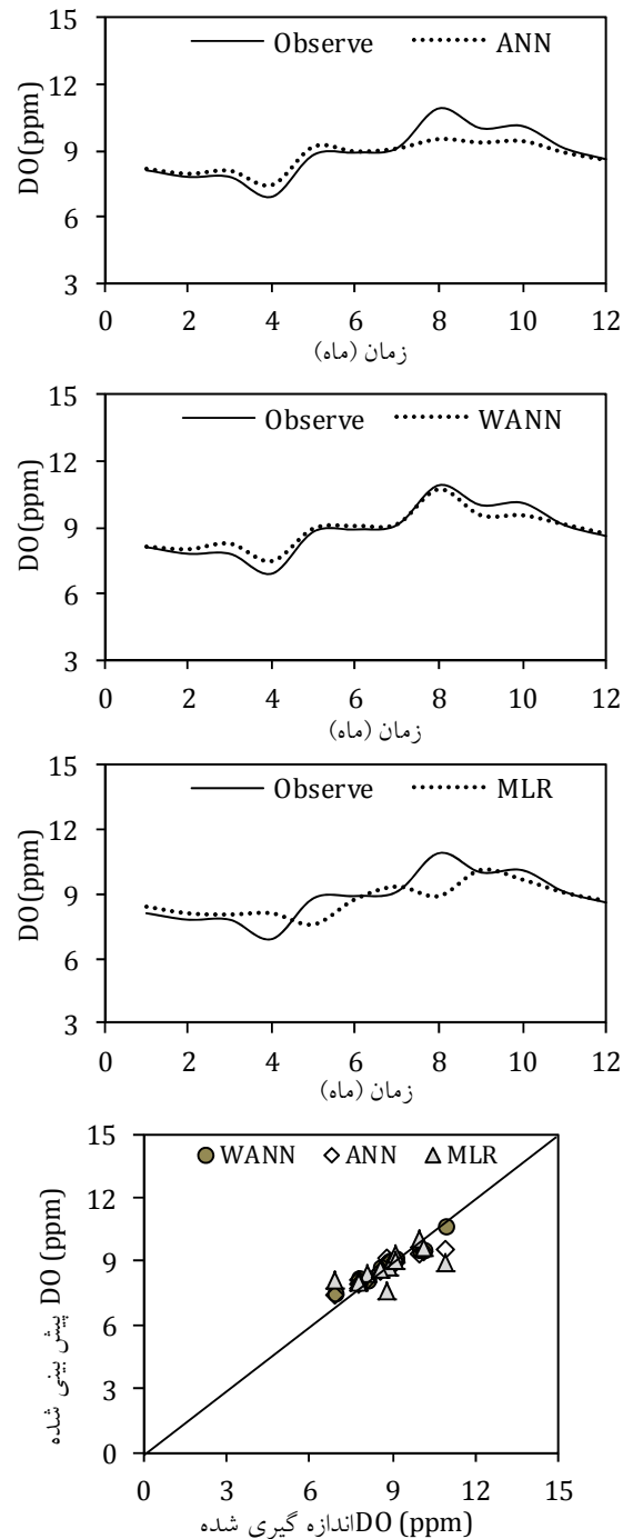
شکل ۸. مقایسه اکسیژن محلول اندازه گیری شده و پیش بینی شده با ANN، WANN و MLR دوره آزمون
