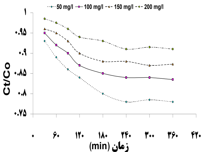
شکل ۱: اثر زمان فرایند و غلظت اولیه راکتیو آبی ۱۹ بر راندمان حذف (جاذب ژئولیت خام و pH=۷)
