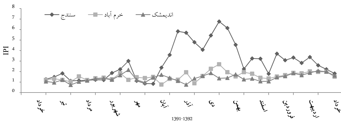
شکل ۶: روند تغییرات شاخص IPI برای فلزات سنگین اندازه‌گیری شده در سه ایستگاه سندج، خرم آباد و اندیمشک
