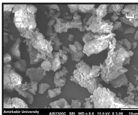
شکل ۷: تصاویر SEM ذرات گرد و غبار در سه ایستگاه سندج (الف)، خرم آباد (ب) و اندیمشک (ج)
