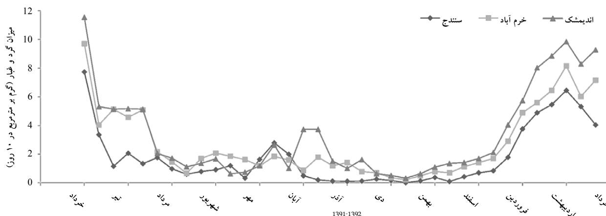
شکل ۲: روند تغییرات میزان ذرات گرد و غبار باریده بر سه شهر سنندج، خرم آباد و اندیمشک در طول دوره نمونه‌برداری ( \text{gr}/\text{m}^2 \cdot 10 \text{ days} )
