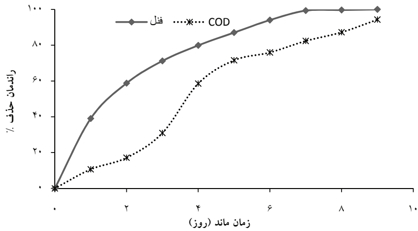
شکل ۳: راندمان تجزیه فصل و حذف COD نسبت به زمان (غلظت اولیه فصل ۵۸۷ mg/L و غلظت اولیه COD ۱۲۳۲ mg/L)
