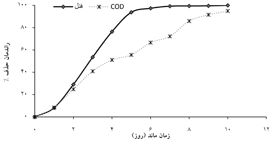
شکل ۴: راندمان تجزیه فصل و حذف COD نسبت به زمان (غلظت اولیه فصل ۹۱۱ mg/L و غلظت اولیه COD ۱۷۷۸ mg/L)
