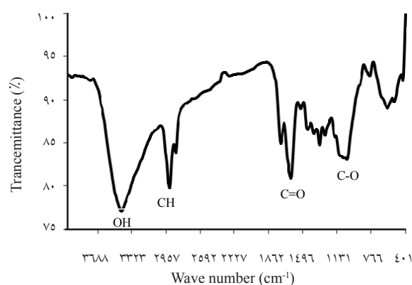
شکل ۲- الف: طول موج FTIR پوست سبز گردو از 4000 تا cm^{-1}
