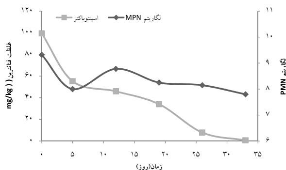
شکل ۱: چگونگی رشد باکتری و حذف فنانتزین توسط اسپتوباکتر sp با غلظت اولیه ۱۰۰ میلی گرم بر کیلوگرم
