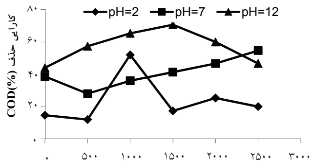
شکل ۵: کارایی سولفات فرو در حذف COD
