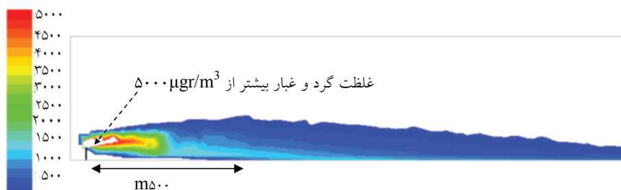
شکل ۴: کانتور غلظت گرد و غبار در مناطقی از صفحه Z=0 که غلظت بیش تر از حد مجاز (۱۵۰ میکروگرم بر متر مکعب) است.
