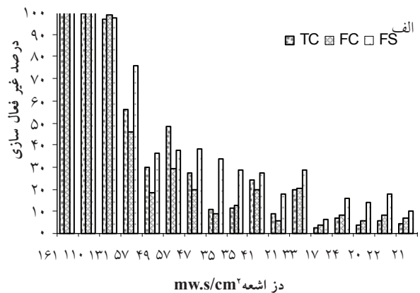
شکل ۴: فعالیت مجدد باکتری های هدف پس از گذردن پساب ثانویه توسط: الف: لامپ کم فشار، ب: لامپ فشار متوسط و ج: تلفیق لامپ های کم فشار و فشار متوسط
