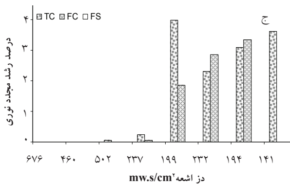
شکل ۴: فعالیت مجدد باکتری های هدف پس از گذردن پساب ثانویه توسط: الف: لامپ کم فشار، ب: لامپ فشار متوسط و ج: تلفیق لامپ های کم فشار و فشار متوسط
