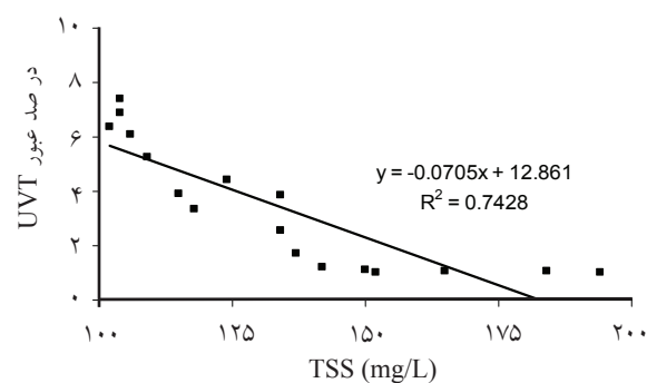
شکل ۲: درصد عبور اشعه UV در مقابل محتوای TSS پساب ثانویه
