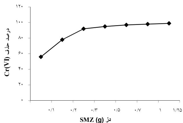
شکل ۲: تأثیر تغییرات دز جاذب SMZ بر کارایی حذف Cr(VI) در C_{Cr} = 1 \text{ mg/L} و pH=7
