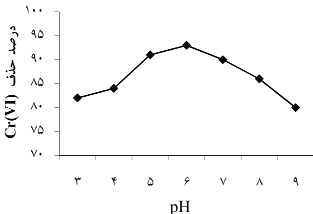
شکل ۳: تأثیر تغییرات pH بر کارایی حذف Cr(VI) در C_{Cr} = 1 \text{ mg/L} و دز 0.3 \text{ gr}
