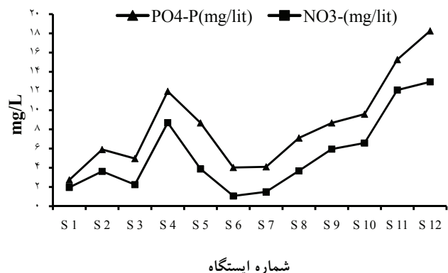
شکل ۵: تغییرات NO_3^- و PO_4^{3-} در رودخانه
