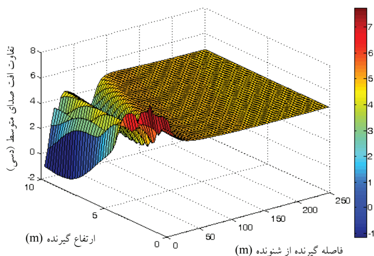
شکل ۶: نمودار سطحی بهبود افت صدا مانع مدل PR۴ نسبت به مانع مدل QR۴ در ۲۰۰
