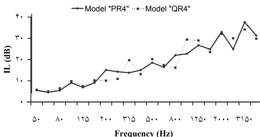
شکل ۳: مقایسه یک مانع T، QRD شکل (مدل QR۴) و یک مانع T، PRD، شکل (مدل PR۴) در نقطه گیرنده (۵۰ و -۵۰) (فرکانس طراحی دو پخش کننده یکسان و ۴۰۰۰ هرتز می‌باشد)
