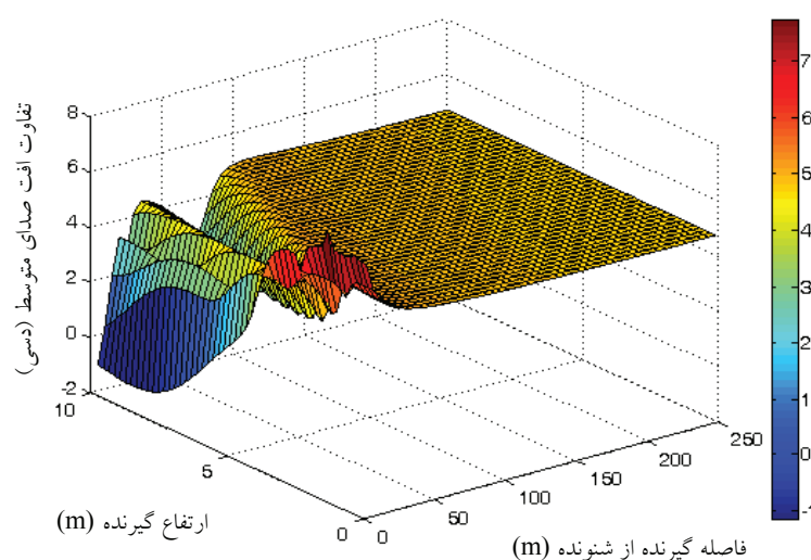
شکل ۶: نمودار سطحی بهبود افت صدا مانع مدل PR4 نسبت به مانع مدل QR4 در 200
