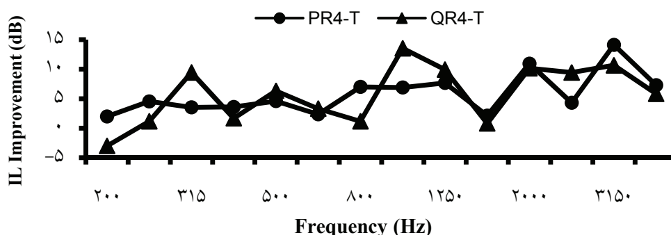
شکل ۴: بهبود افت صدای حاصل از مانع مدل PR۴ و QR۴ نسبت به مانع مرجع در نقطه گیرنده (۵۰ و -۵۰)
