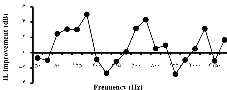
شکل ۸: بهبود افت صدای حاصل از به کارگیری وایریش با مقاومت r=1/5 Rayls در مانع مدل PR۴ در نقطه گیرنده (۵۰ و ۵۰۰)
