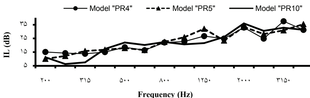
شکل ۷: اثر PRD با فرکانس‌های طراحی متفاوت در مانع T شکل نقطه گیرنده (۵۰ و ۵۰۰)
