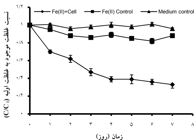
شکل ۲: احیا میکربی نیترات در حضور Fe 2+ به عنوان منبع الکترون در دمای ۳۰ درجه سانتی گراد (مقادیر نشان داده شده در شکل میانگین و انحراف معیارهای مربوط به هر میانگین در هر نقطه می باشد)
