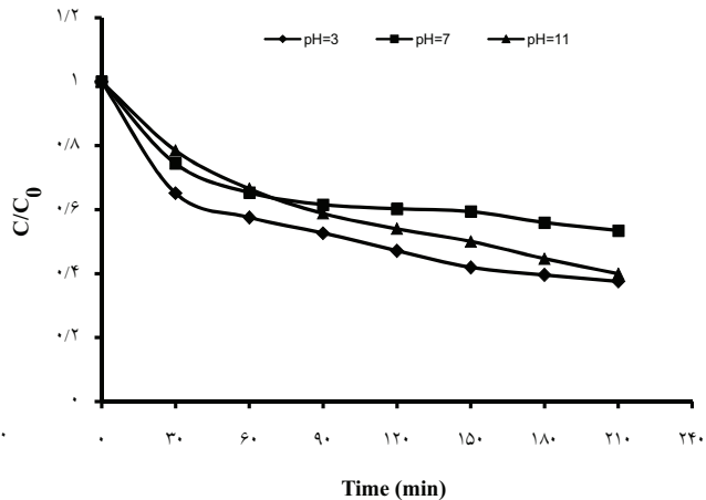
شکل ۵: تاثیر pH در تجزیه فتوکاتالیستی فنل: C_0=100 \text{ mg/L} ، \text{Fe}^{3+}-\text{TiO}_2=0/5 \text{ g/L} ، C_0 و C غلظت فنل به ترتیب در زمان های صفر و t.
