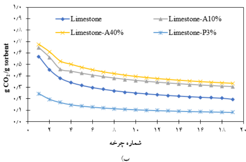
نمودار ۴- تاثیر غلظت‌های مختلف اسید در میزان جذب \text{CO}_2 (الف) میزان تبدیل، (ب) ظرفیت جذب جاذب‌ها
