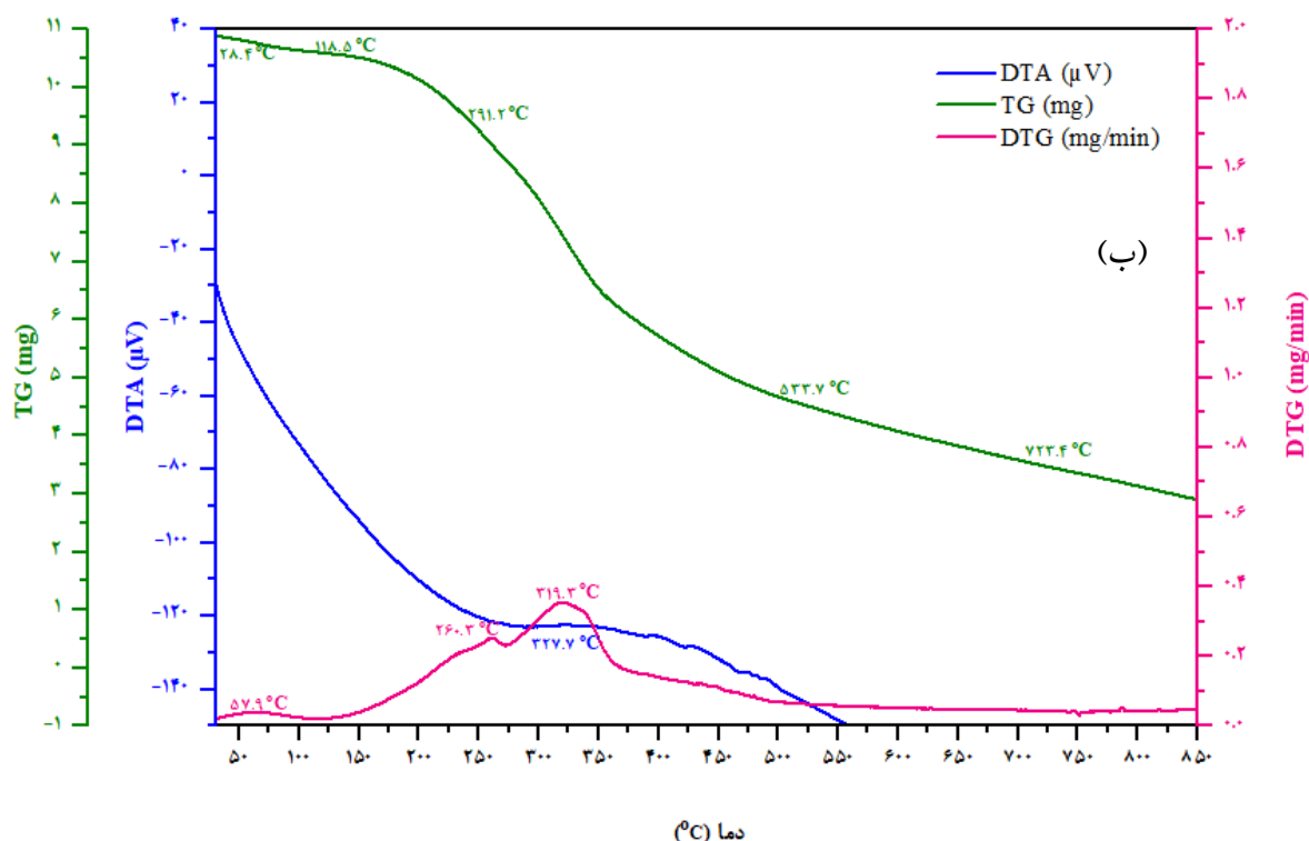
ادامه نمودار ۳- منحنی آنالیز توزین حرارتی الف (SCG و ب) هیدروچار حاصله در شرایط بهینه ( 235^{\circ}\text{C} , ۱۸۰ min و نسبت L:S:۸:۱)
