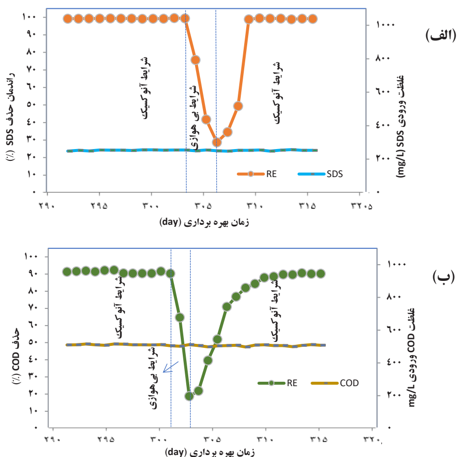
نمودار ۴- اثر عدم حضور نیترات در حذف SDS (الف) و COD (ب) در غلظت ۲۵۰ mg/L SDS و HRT=4\text{ h}
