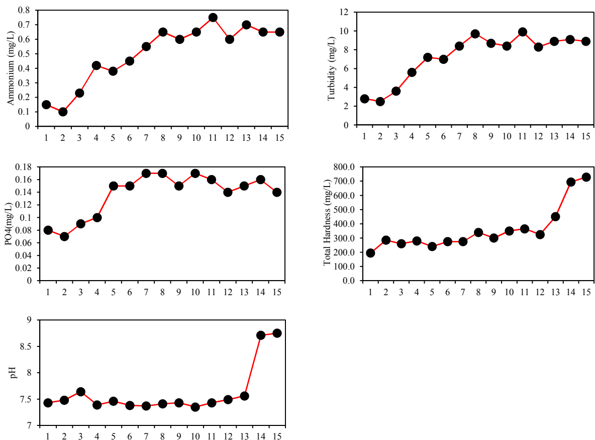
ادامه نمودار ۱- روند تغییرات پارامترهای کیفیت آب در ایستگاه‌های مورد مطالعه از بالادست به پایین دست رودخانه
