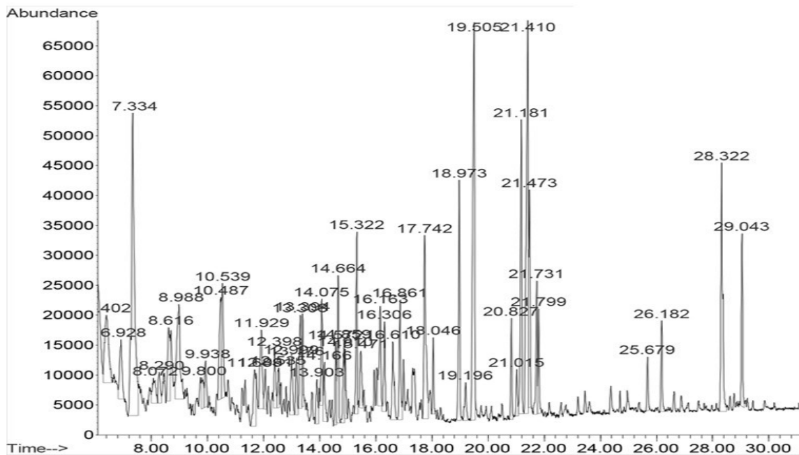
نمودار ۱- نمودار کروماتوگرام سموم در نمونه‌های شیر دارای سم
