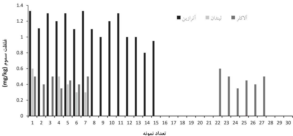
نمودار ۲- غلظت سموم آلاکلر، لیندان و آترازین در نمونه‌های شیر خام
