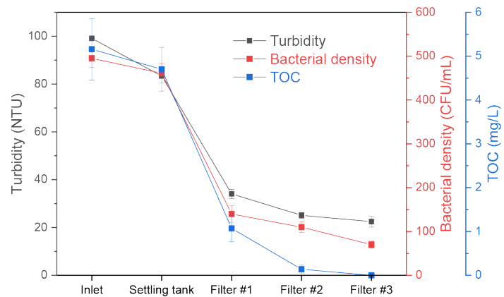
نمودار ۶- میانگین حذف TOC و عوامل میکروبی در واحد فیلتر اسفنجی بافل دار (کدورت ۱۰۰ NTU و بار سطحی ۱۰ m/h)
