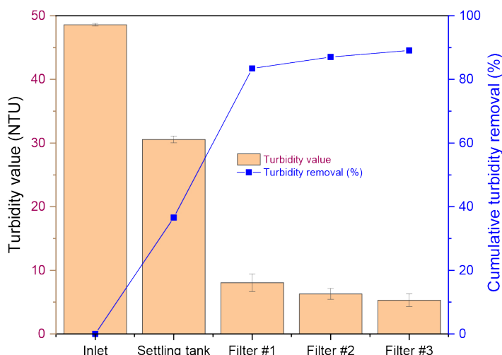
نمودار ۲- میانگین حذف کدورت ۵۰ NTU در فیلترهای اسفنجی بافل دار در بار سطحی ۱۰ m/h
