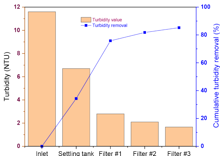
نمودار ۱- میانگین حذف کدورت ۱۰ NTU در فیلترهای اسفنجی بافل دار در بار سطحی ۱۰ m/h
