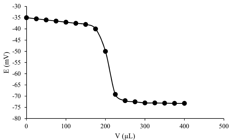
شکل ۴- منحنی تیتراسیون محلول 10^{-6} \text{ M} نیترات کادمیم با محلول 10^{-4} \text{ M} EDTA
