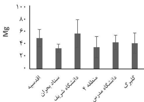
ادامه نمودار ۳- درصد فاکتور غنی شدگی (EF (%)) عناصر Cu, Zn, Ni, Pb, Cr, Co, Fe, Mn, Na و Mg در گل‌سنگ R. sinensis در ایستگاه‌های مختلف کلانشهر تهران
