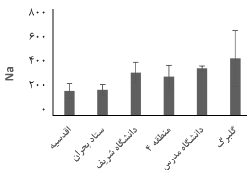
ادامه نمودار ۳- درصد فاکتور غنی شدگی (EF (%)) عناصر Cu, Zn, Ni, Pb, Cr, Co, Fe, Mn, Na و Mg در گل‌سنگ R. sinensis در ایستگاه‌های مختلف کلانشهر تهران
