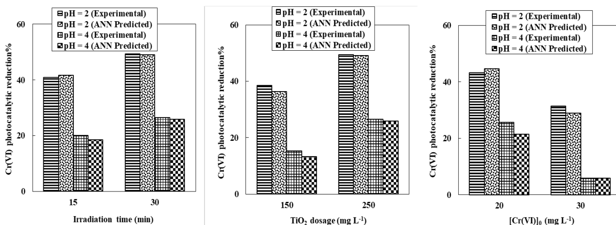
نمودار ۴- تاثیر غلظت اولیه Cr(VI) و pH (الف)، مقدار کاتالیزور TiO_2 و pH (ب) و زمان تابش نور و pH (ج) بر روی درصد احیاء Cr(VI) تحت شرایط Time = 15 \text{ min} , [TiO_2]_0 = 150 \text{ mg/L} ، (الف)، Time = 30 \text{ min} , [Cr(VI)]_0 = 30 \text{ mg/L} و (ب) و [TiO_2]_0 = 250 \text{ mg/L} , [Cr(VI)]_0 = 30 \text{ mg/L} (ج).
