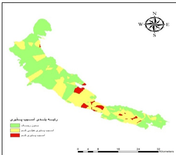
شکل ۱- نقشه پهنه بندی آسیب پذیری محدوده دشت با روش دراستیک
