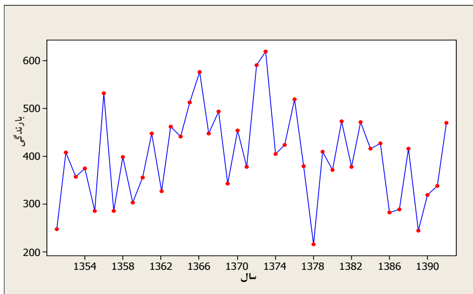
نمودار ۱- نمودار سری زمانی بارندگی سالیانه ایستگاه باران‌سنجی ماهیدشت
