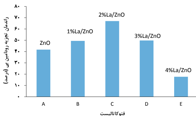
نمودار ۱- اثر مقدار لانتانیم روی راندمان تجزیه فتوکاتالیستی رودامین بی (غلظت اولیه محلول رودامین 4.79 \text{ mg/L} ، \text{pH}=9 ، مقدار فتوکاتالیست 1/25 \text{ g/L} ، زمان 120 \text{ min} )
