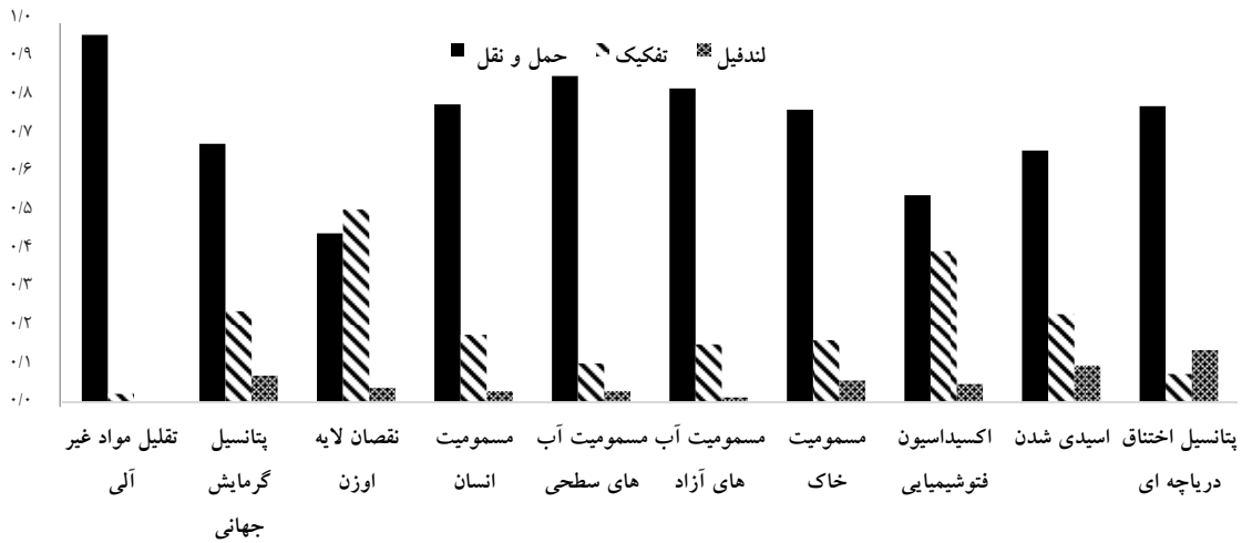
نمودار ۵- سهم هر یک از فرایندها در انتشار آلاینده‌های زیستی زیرسامانه لندفیل جهانی
